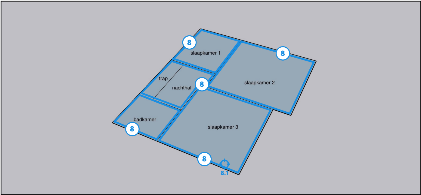
Legende van plan 1.9: Grondplan 1e verdieping c
